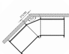
Esquina externa 90°
