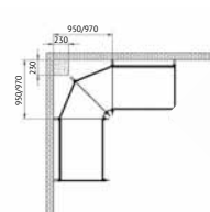
Esquina interna 90°
