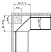
Esquina interna 45° + 45°
