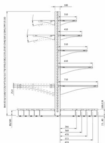
Panel trasero central. Tipo 2
