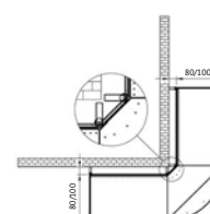
Esquina interna 45°
